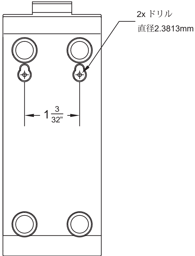
充電クレードル 壁取り付けテンプレート スケール 1.000
