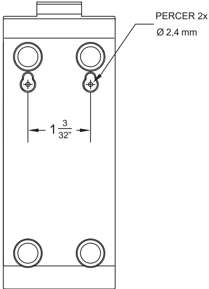
GABARIT POUR LA FIXATION MURALE DU SOCLE DE CHARGE ÉCHELLE 1/1000
