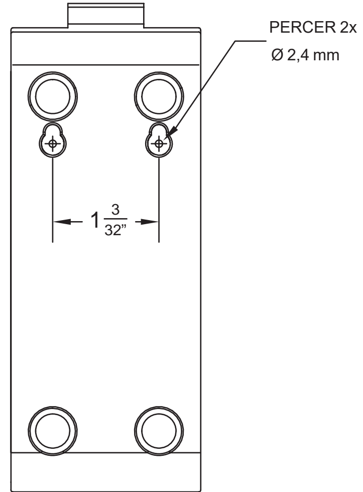
GABARIT POUR LA FIXATION MURALE DU SOCLE DE CHARGE ÉCHELLE 1/1000
